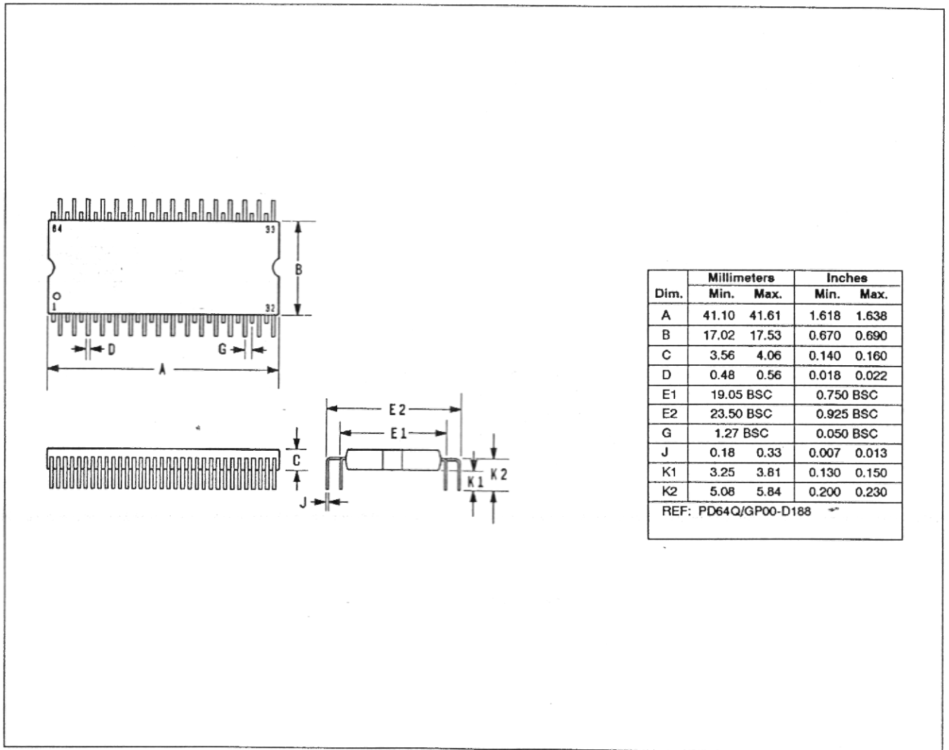
64-Pin QUIP
